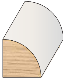
PROFILE # FJP2222Q DIMENSION 1 1/16" x 1 1/16"
