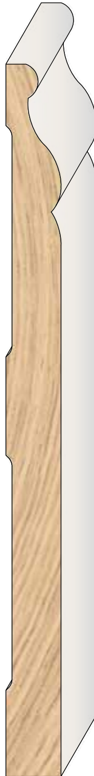
PROFILE # PFP18232CB DIMENSION 9/16" x 7 1/4" x 16'
